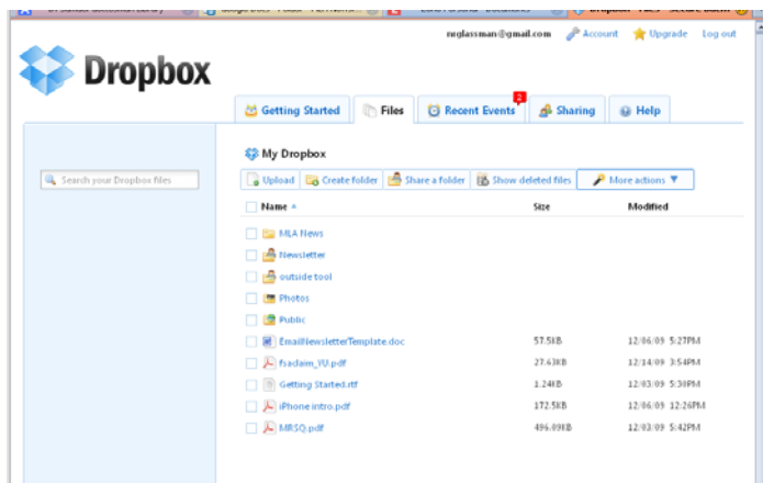
Dropbox
