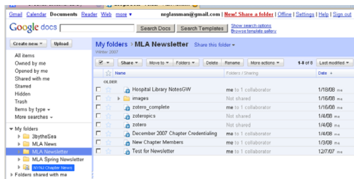
Google Docs
